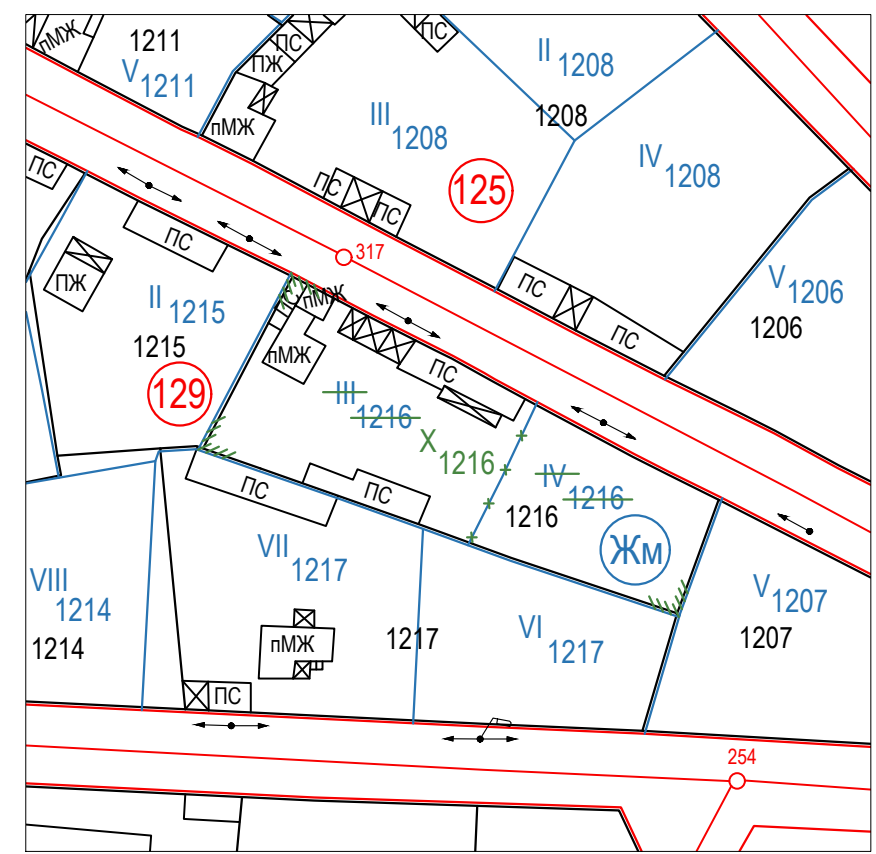
ПЛАН ЗА РЕГУЛАЦИЯ М 1:1000
